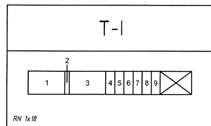
widok rozdzielnic
